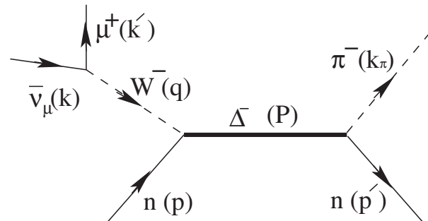
FIG. 3. Feynman diagram.
