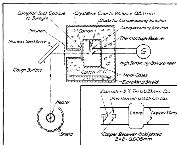
Fig. 1. Apparatus.
